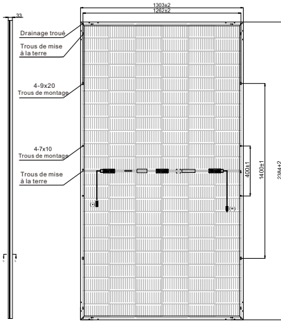
Dimensions du module PV Unité: mm
